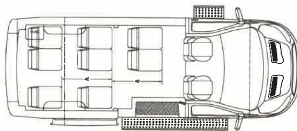
9-PASSENGER
